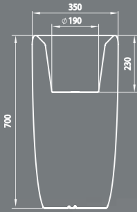
9712 FLOWERPOT ↑ 70 cm ∅ 35 cm 1 x E27, max 60W
