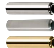
■ Door stop on wall Dveřní doraz na zed' Wandtürstopper Дверной упор настенный 18 x 18 x 80 mm 101218022 chrome / chrom 101218025 stainless matt / nerez 101218027 brass / mosaz
